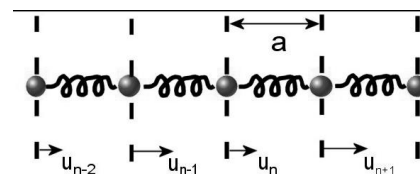
Figur 1. Atomi i ein krystallstruktur kann upp til andre orden modellerast som eit system av kulor og fjører.
