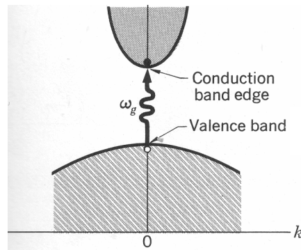
Figur 2. Bandstrukturen i ein halvleidar.
