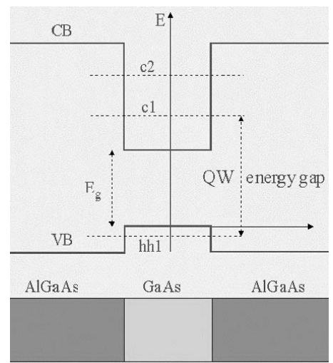
Figur 2. Potensialbrunn dana i det tvo material med kvar sine bandstrukturar, AlGaAs og GaAs, vert slutta saman. Som me kann sjå vert det i GaAs-sjiktet dana ein potensialbrunn der elektron og hol let seg fanga. Når dei rekombinerar, sender dei ut foton med energien som svarar til bandgapet i GaAs.
