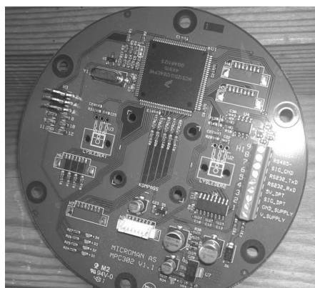
Nytt produkt: Det runde kortet er bruka i eit instrument som mæler bylgjehøgdi, temperatur, ljøs og straum i sjøen. Det er sett i hop av ytemonterte krinsar (Foto: Kolbjørn Tvedt).
