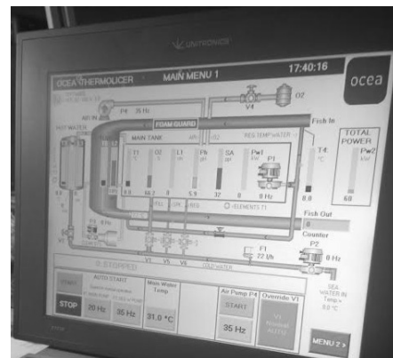
Innovasjonen gjeng vidare: Her er me på laboratoriet og ser eit PLC-prosesserprogram til ein avlusar for laks som Microman held på å utvikla no for tida (Foto: Kolbjørn Tvedt).
